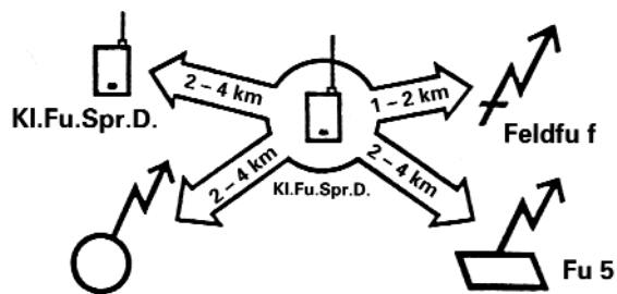
Рис. 8. Kl.Fu.Spr.d в системе радиосредств Вермахта
